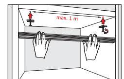
Clemele pentru profilele Line XL.
