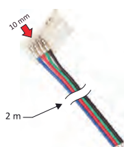
76. MICRO CONECTOR PENTRU BANDĂ LED RGB 10MM, CABLU 2M, CAPETE GALVANIZATE
