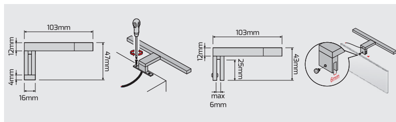
Două opțiuni de montaj, un singur produs
