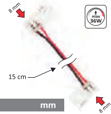
70. MICRO CONECTOR PENTRU BANDĂ LED 8 MM, CABLU 0.15 M, CU MINIMUFĂ LA AMBELE CAPETE
