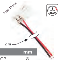
68. MICRO CONECTOR PENTRU BANDĂ LED 8 SAU 10 MM, CABLU 2 M, CAPETE GALVANIZATE
